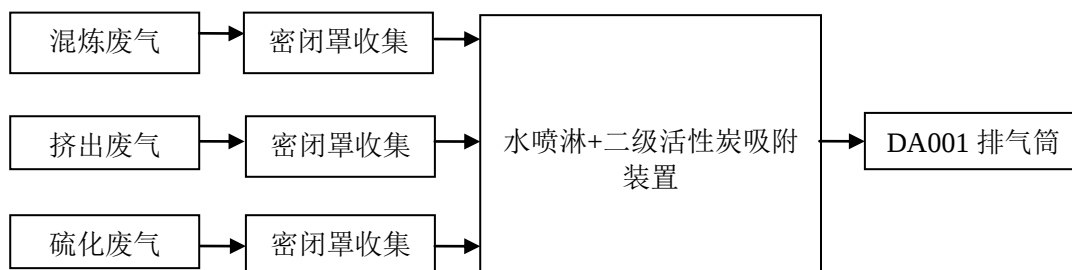
图 4-1 废气处理措施图
