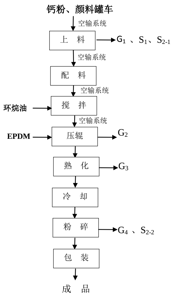
图 2-1 现有项目生产工艺流程及产污环节图
