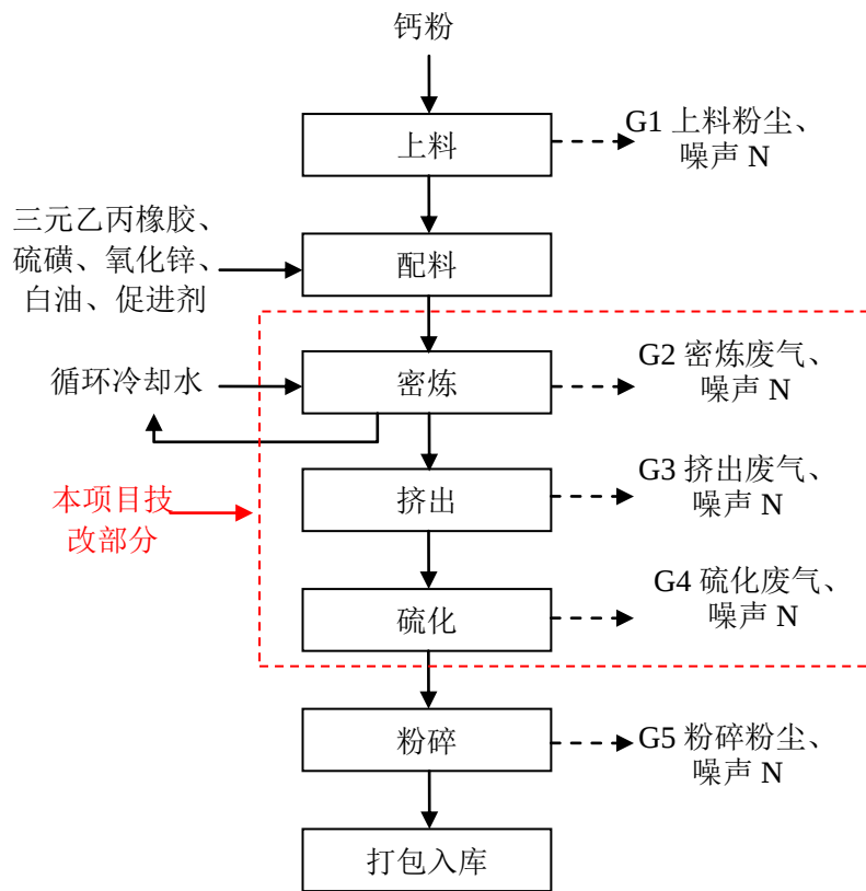
图 2-2 本项目生产工艺流程及产污环节图
