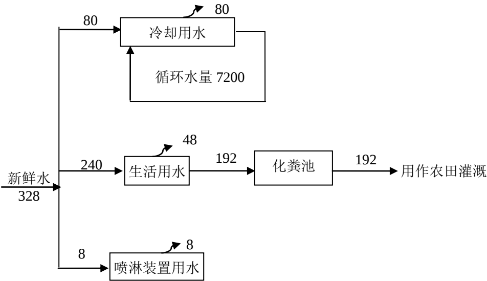
图 2-1 技改实施后全厂水平衡图
