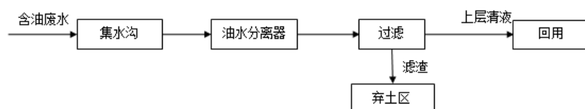
图 5-3 含油废水处理工艺流程图
