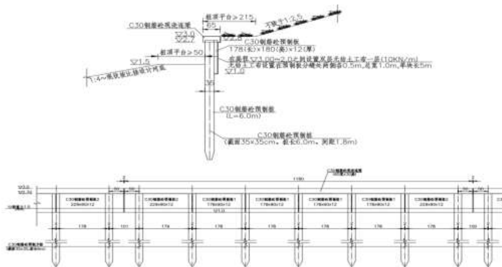
图 2-19 插板桩护岸设计断面
