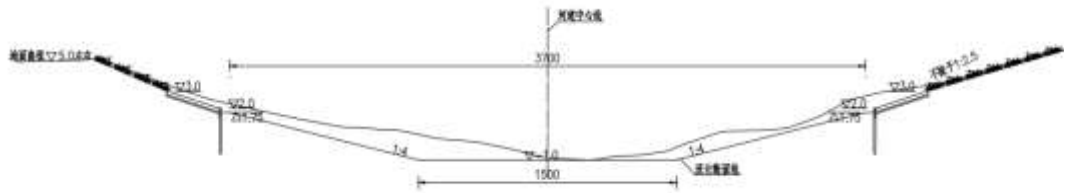
图 2-11 桩号 6+200~7+250 段河道设计断面
