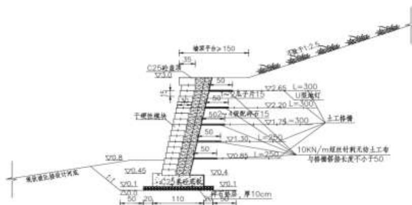
图 2-20 模块墙护岸设计断面
