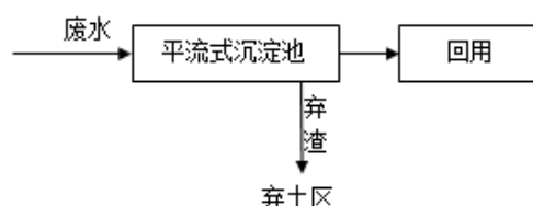
图 5-1 施工场地的泥浆废水处理流程图
