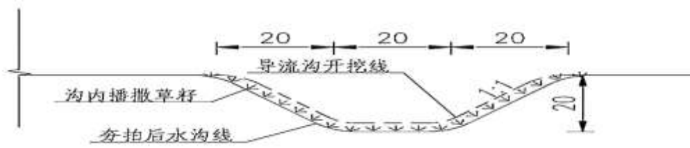
图 2-23 植草导流沟做法图
