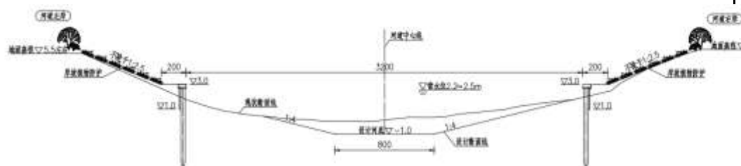
图 2-5 桩号 3+200~3+600 段河道设计断面
