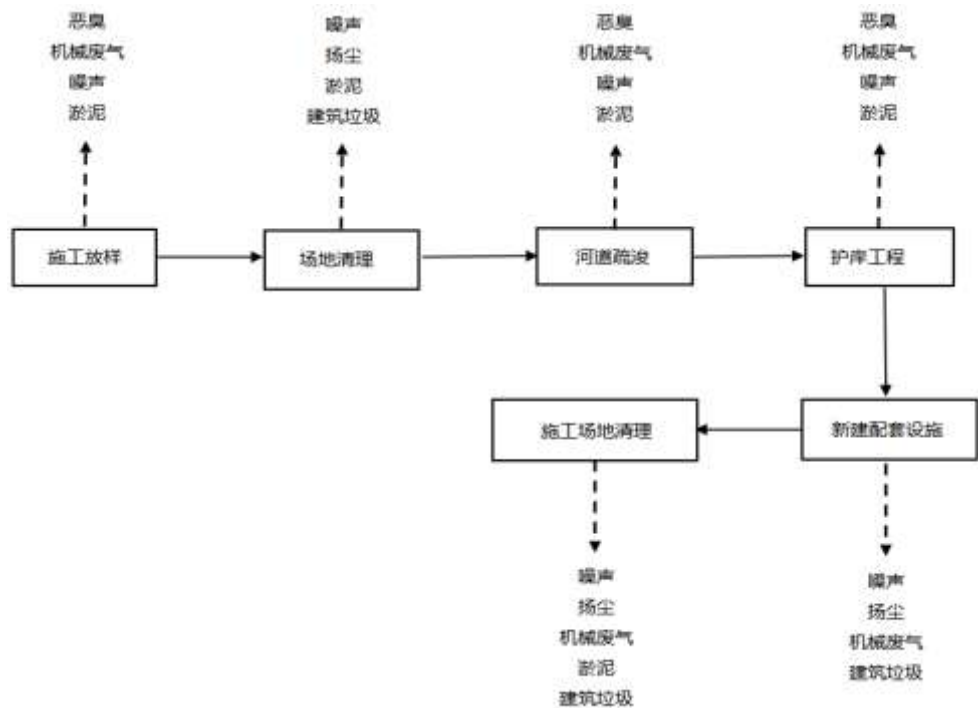
图 2-2 工艺流程图
