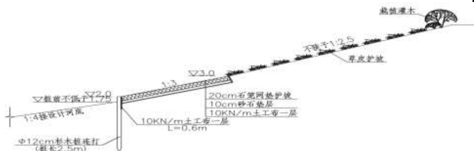
图 2-16 木桩（2.5m）+格宾石笼护坡设计断面
