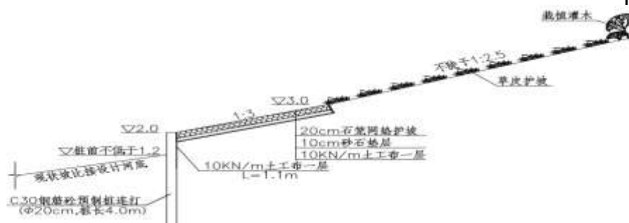
图 2-18 仿木桩（4.0m）+格宾石笼护坡设计断面
