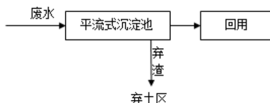
图 5-2 混凝土拌和系统冲洗废水处理流程图
