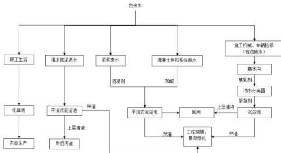
图 4-1 施工期废水流向图
