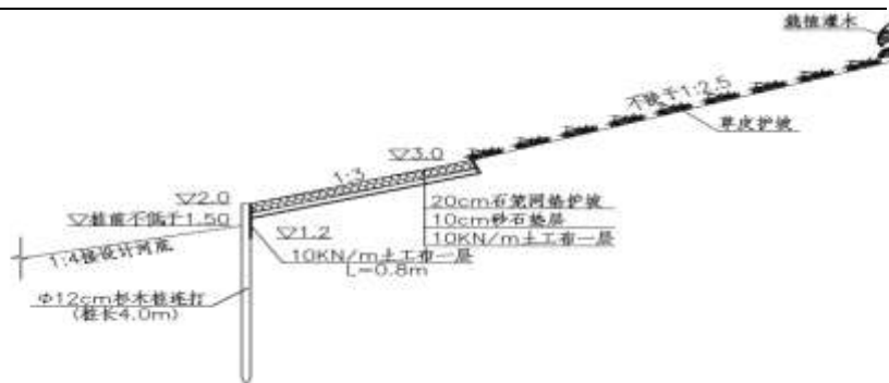
图 2-17 木桩（4.0m）+格宾石笼护坡设计断面
