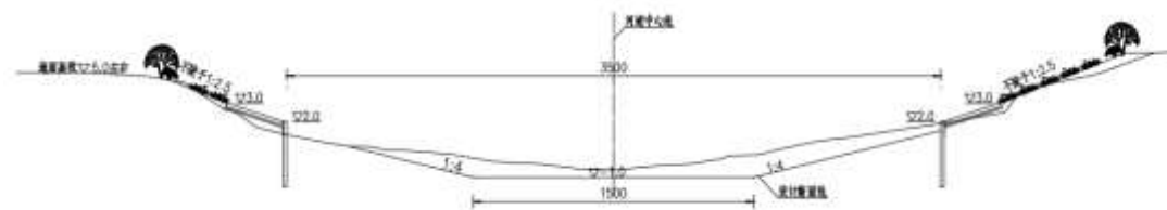
图 2-10 桩号 6+000~6+200 段河道设计断面
