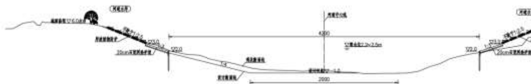
图 2-15 中宣堡港~纪沟桥段河道设计断面
