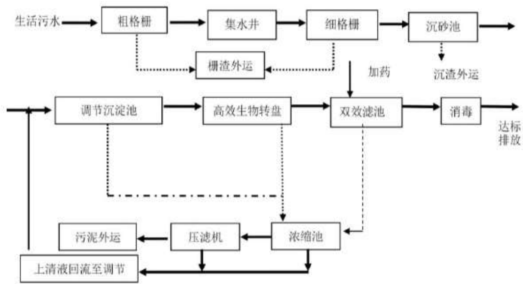
图 4-2 荻垛镇污水处理厂污水处理工艺流程图
