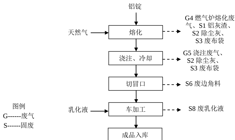
图 2-3 工字轮、电动车减振铝筒生产工艺流程及产污环节图
