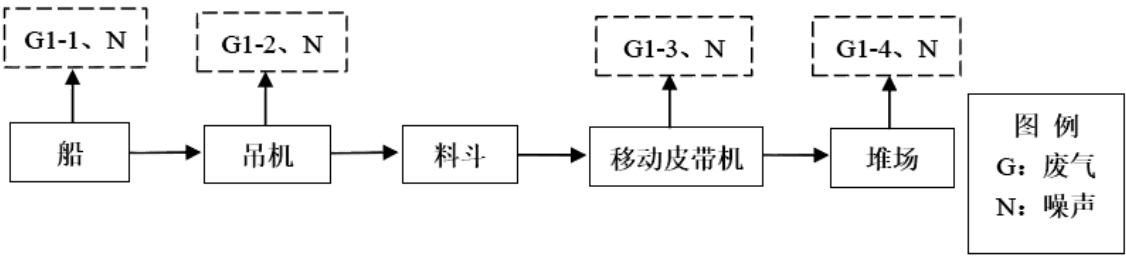
图 2-3 现有项目生产工艺流程及产污环节图
