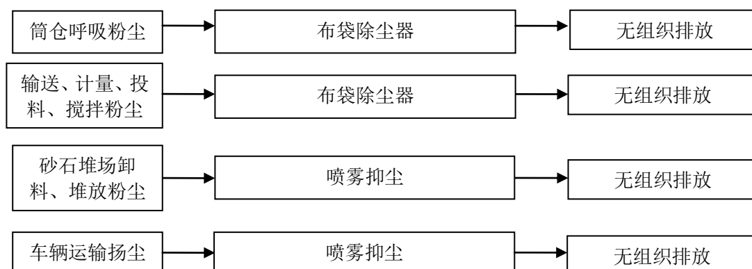
图 4-1 废气处理措施图
