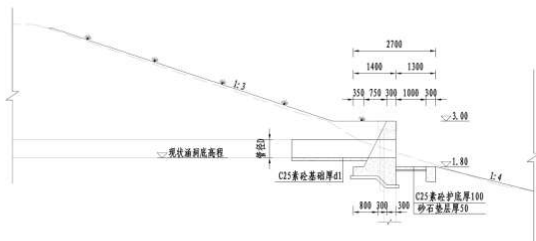
图 2-7 排水口典型断面一
