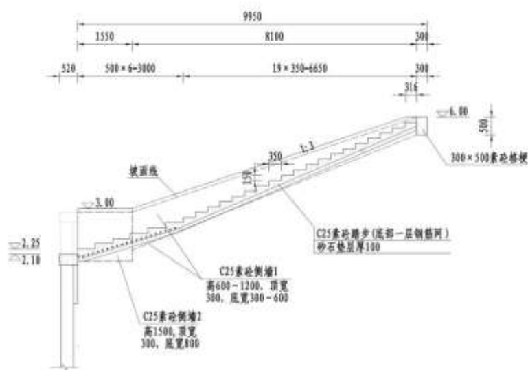
图 2-6 下河踏步纵剖面图
