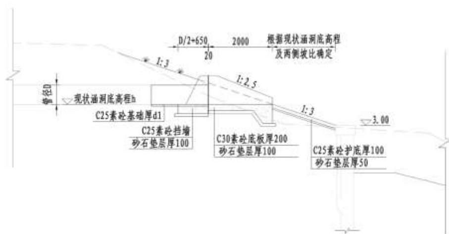
图 2-8 排水口典型断面二
