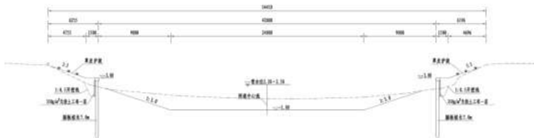
图 2-5 插板桩护岸典型断面
