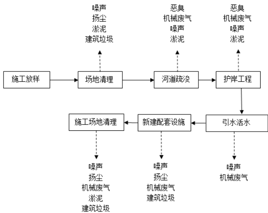
图 2-3 生产河（姜堰区）主体工艺流程图
