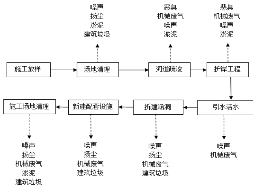
图 2-1 小港河主体工艺流程图
