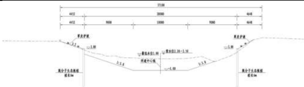
图 2-4 高分子聚合物板桩断面图
