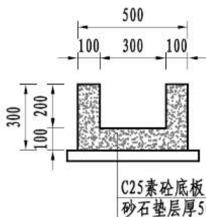
图 2-9 岸坡排水沟结构设计图
