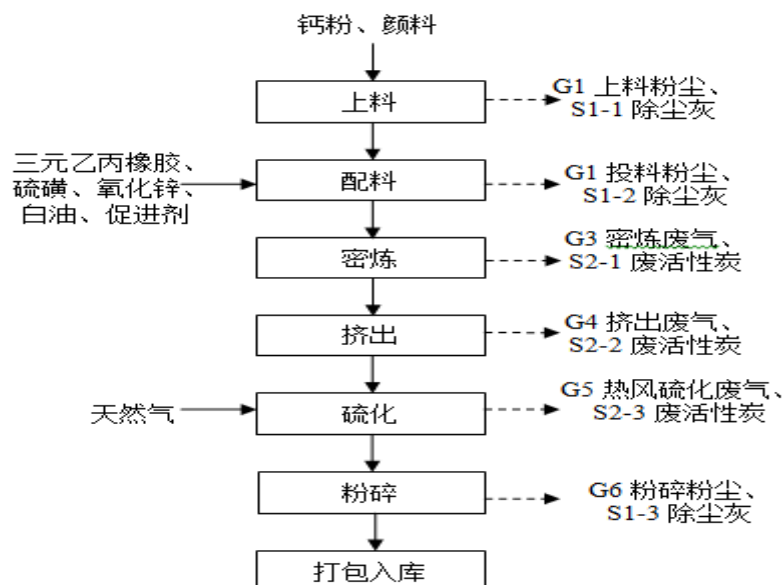
图 2-2 原有项目生产流程及产污环节图
