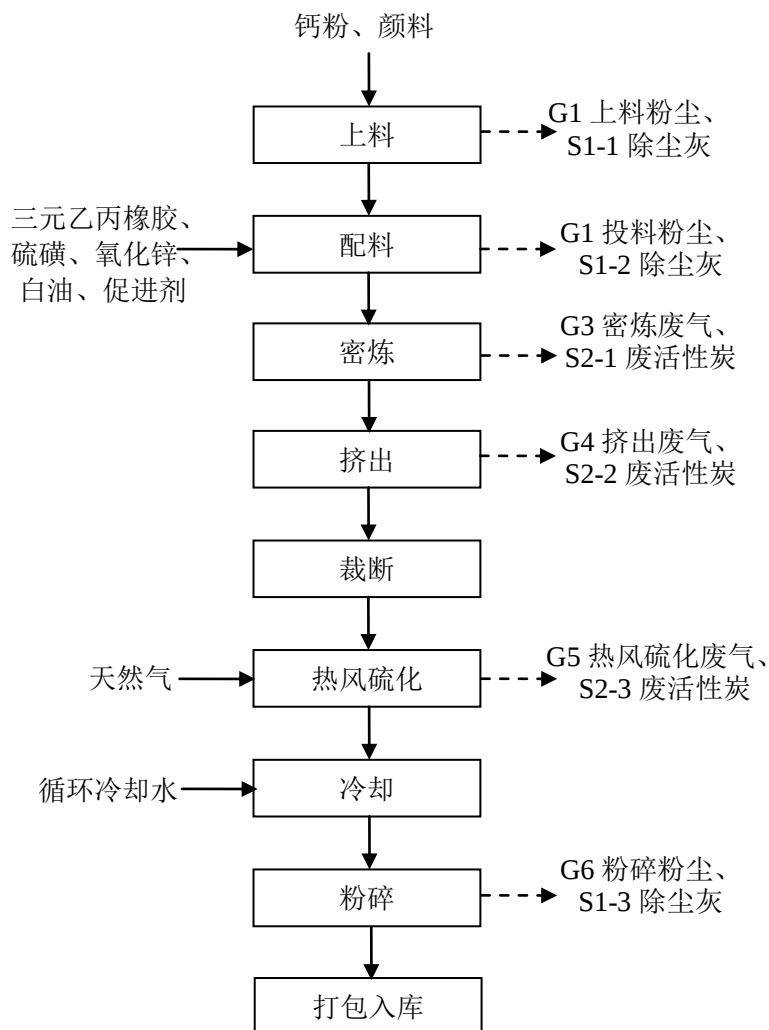
图 2-1 本项目生产工艺流程及产污环节图
