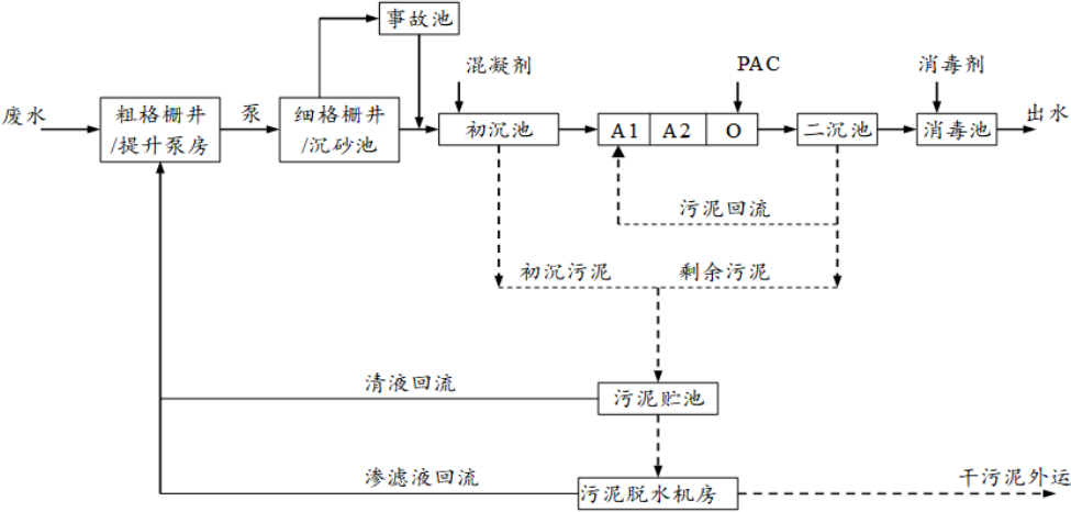
图 7-1 九龙镇污水处理厂工艺流程图
