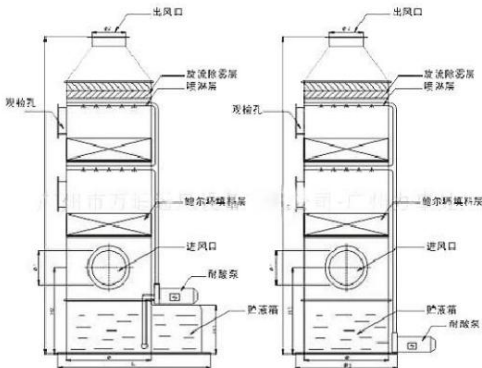
图 5-4 碱喷淋塔废气处理技术原理示意图
