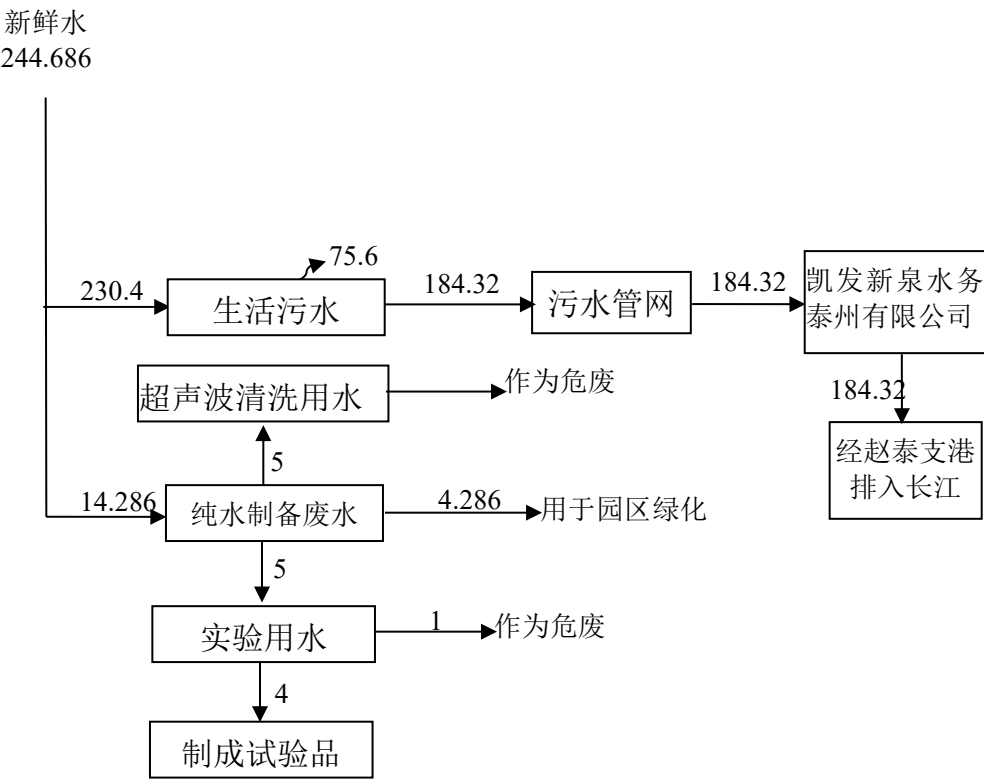
图 5-3 项目用水平衡图 单位：m³/a
