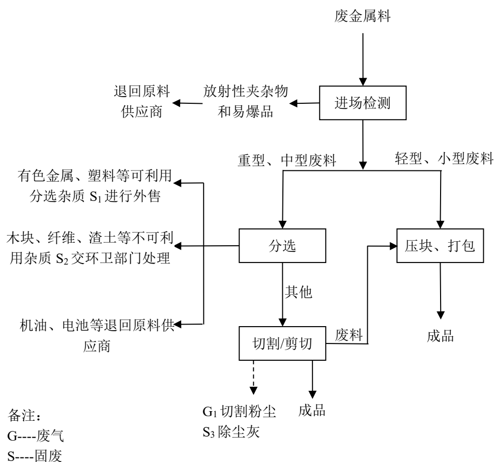
图 5-1 废钢加工生产工艺流程及产污环节图
