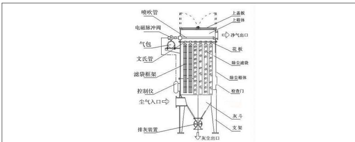
图 5-4 布袋除尘器示意图
