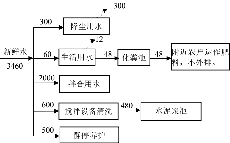
图 5-3 项目用水平衡图 单位：m³/a
