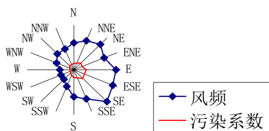
图 2-1 风向玫瑰图
