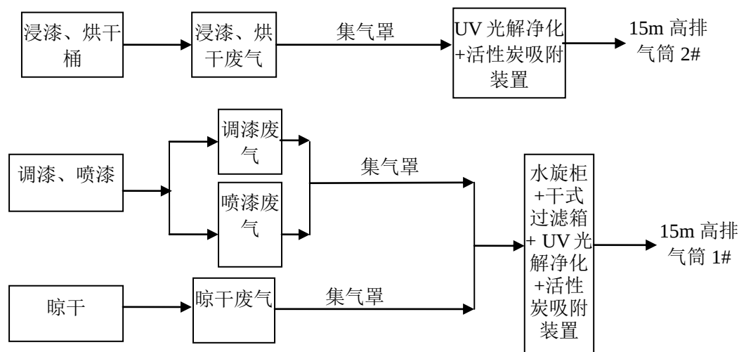
图 5-4 各类有组织废气收集、处理走向图
