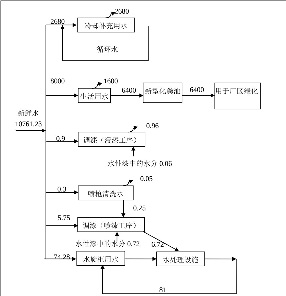
图 5-3 技改后全厂用水平衡图 单位 \text{m}^3/\text{a}
