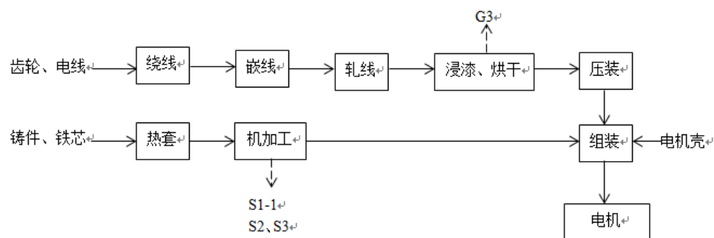
图 5-2 电机加工流程及产污环节图
