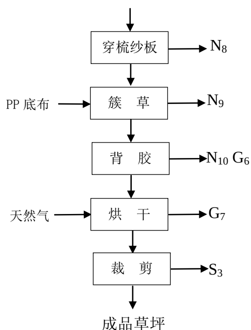
图 5-3 人造草坪生产工艺流程及产污环节图
