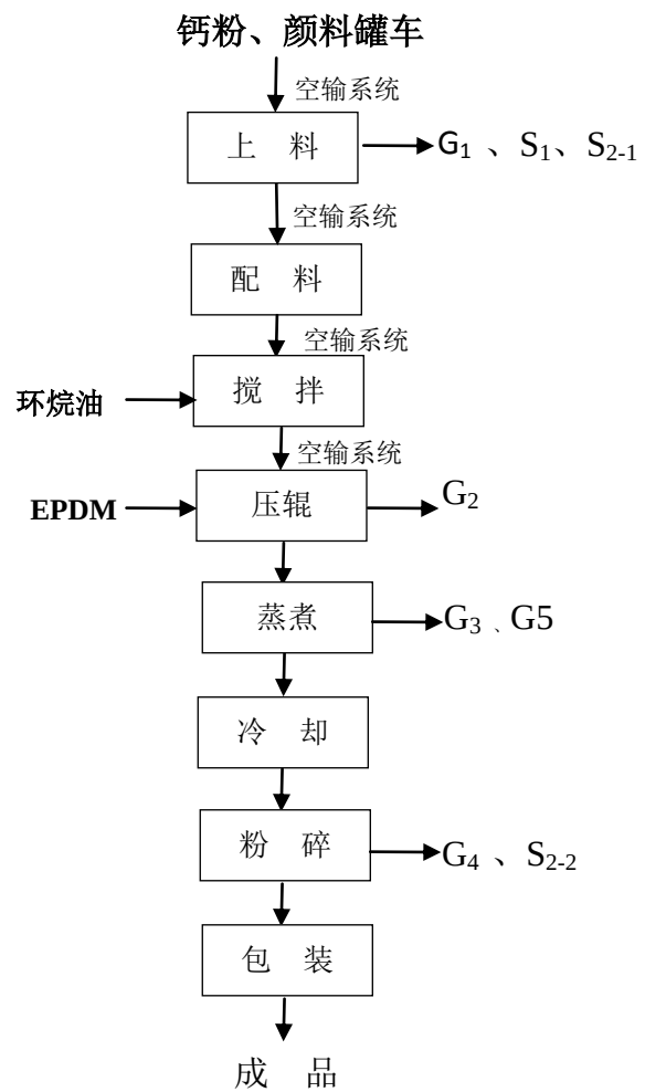
图 5-1 体育材料生产工艺流程及产污环节
