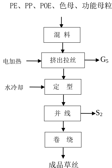
图 5-2 人造草丝生产工艺流程及产污环节图
