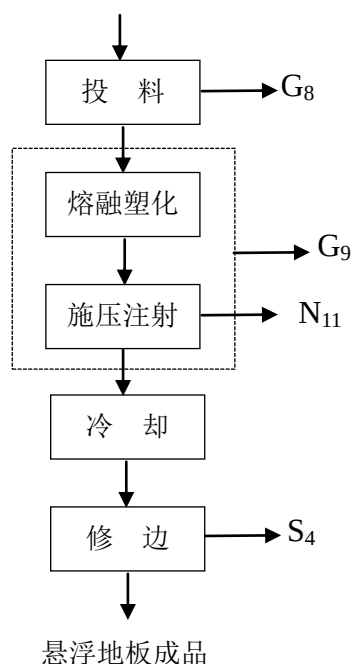
图 5-4 悬浮地板生产工艺流程及产污环节图
