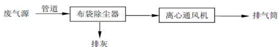
图 5-4 布袋除尘器工艺流程图
