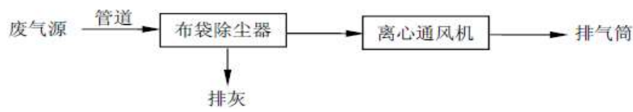
图 5-4 布袋除尘器工艺流程图
